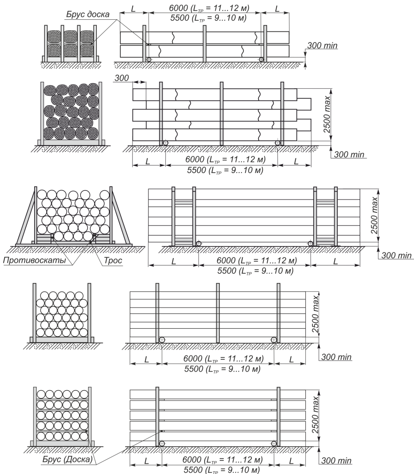
Рисунок 6 - Схемы укладки буровых труб
